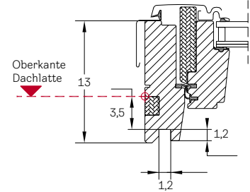
Vertiefter Einbau
